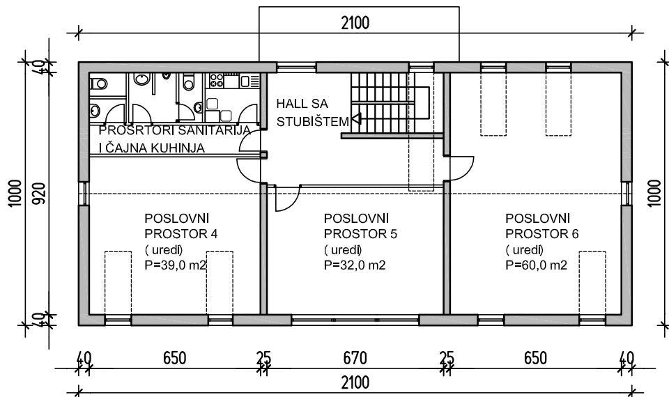
TLOCRT 1. KATA
