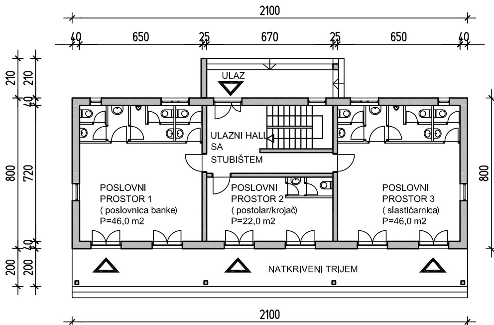
TLOCRT PRIZEMLJA
